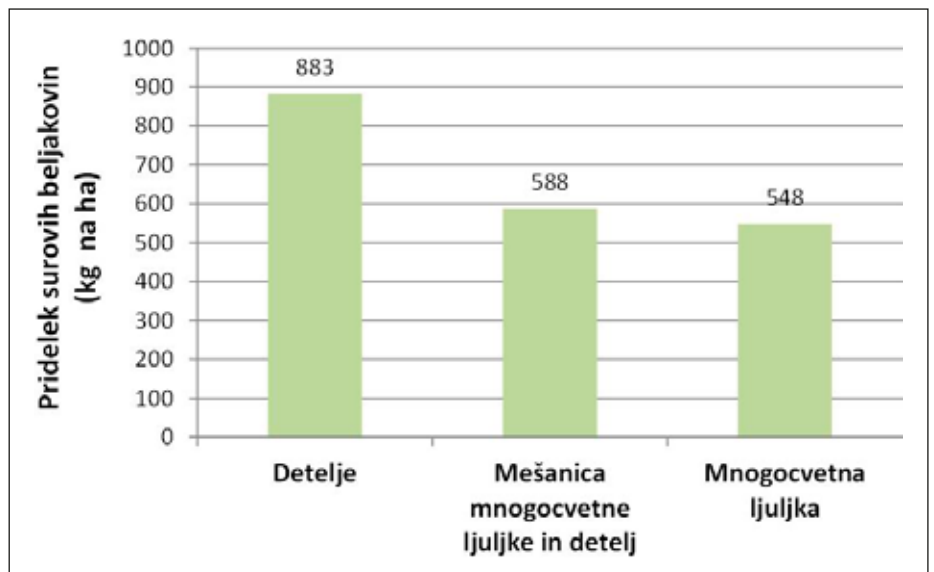
Slika 2. Povprečni pridelki surovih beljakovin z mešanico detelj, mešanico mnogocvetne ljuljke z deteljami in mnogocvetne ljuljke v čisti setvi.
