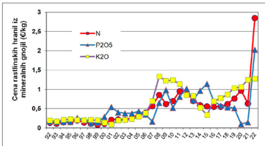
Slika 1. Cene rastlinskih hranil iz mineralnih gnojil (brez DDV) v obdobju 1992–2022 (vir: Moljk, 2022 in proizvodbe na trgu). Ocene za pomlad 2022 so zaradi velikih dnevnih nihanj in velikih razlik med ponudniki nezanesljive.
