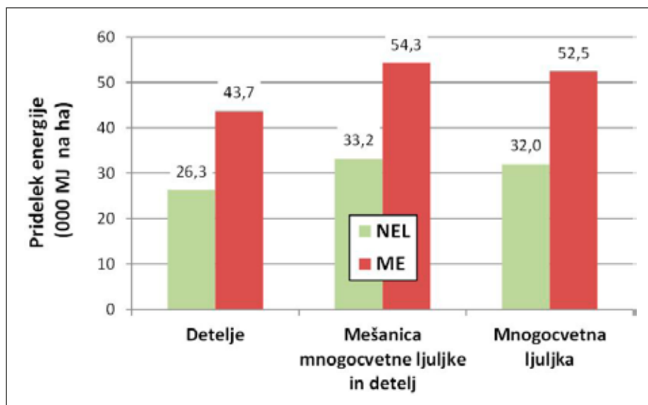
Slika 1. Povprečni pridelki neto energije za laktacijo (NEL) in presnovljive energije (ME) z mešanico detelj, mešanico mnogocvetne ljuljke z deteljami in mnogocvetne ljuljke v čisti setvi.
