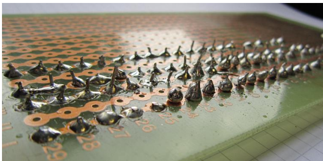
Primer nepravilnega spajkanja, nepravilni spoji.
