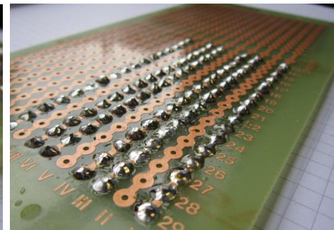
Pogled na stran spajkanja, dobri spoji.
