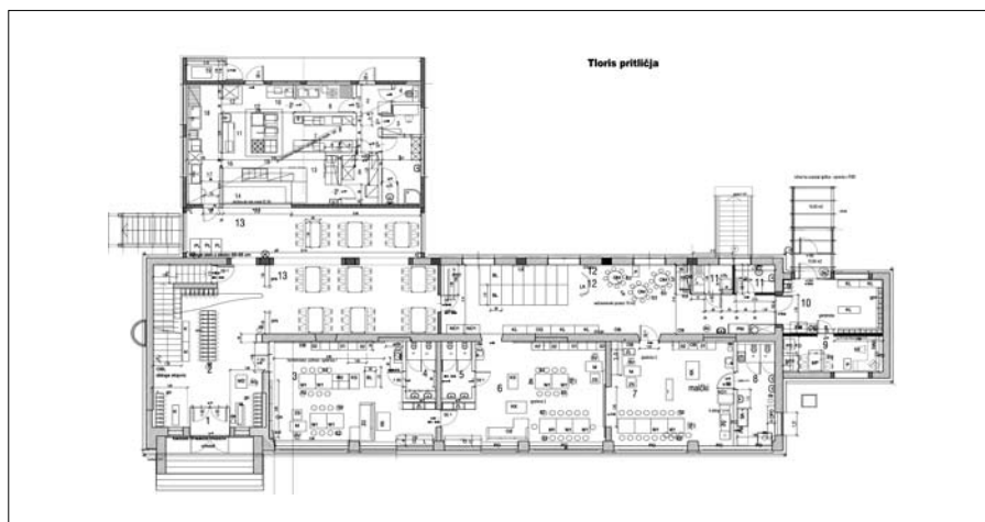
Tloris pritličja, arhitekt Borut Simič
