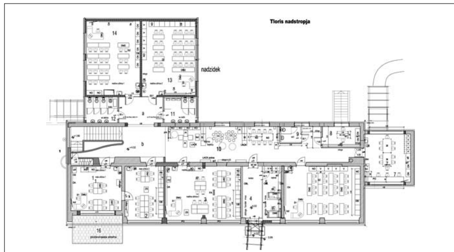
Tloris nadstropja, arhitekt Borut Simič
