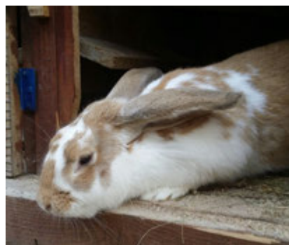
Mešani burgundec
