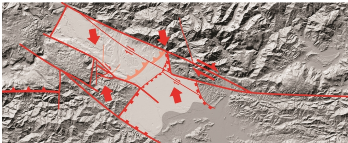
Slika 47: Mehanizem rotacije Rovnika in desnozmčne reaktivacije Nemiljske tektonske cone.
