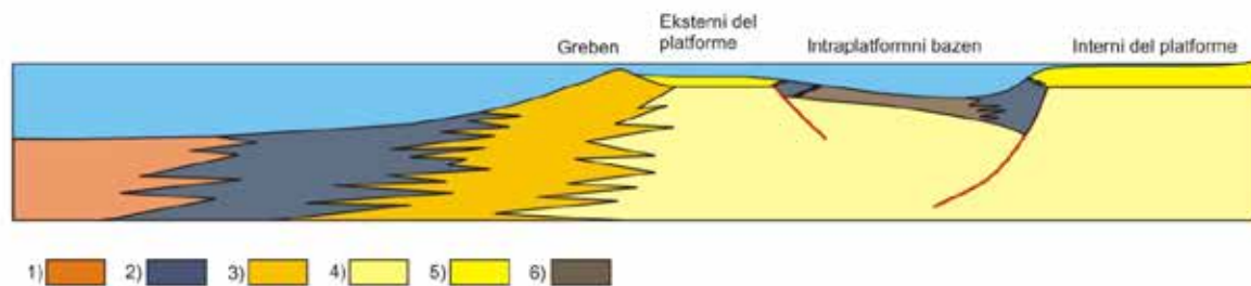
Slika 23: Shematski prikaz strukture karbonatne platforme, kakršne so pri nas obstajale v Tetidi v času mezozoika. 1) globokomorski sedimenti, 2) pobočni sedimenti, 3) greben, 4) platformne karbonatne kamnine, 5) karbonati zunanjega dela platforme, 6) globjevodni karbonati intraplatformnih bazenov. Po Žalohar in Celarc (2010).
