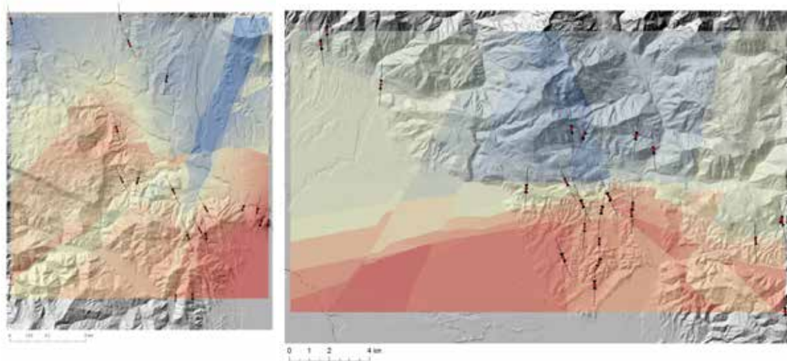
Slika 40: Paleonapetostna karta ozemlja za fazo kompresije NW-SE do N-S interpolirana z metodo Kriging. a) zahodni del ozemlja med Kropo in Kranjem; b) vzhodni del ozemlja v okolici Kamnika. Rdeča barva predstavlja pozitivno vrednost relativne vertikalne deformacije, modra barva pa predstavlja negativno vrednost relativne vertikalne deformacije.
