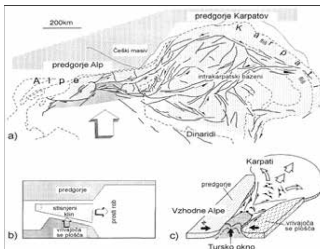
Slika 18: Model lateralne ekstruzije v Vzhodnih Alpah (po Ratsbacher et al., 1991a, b). a) pregledna tektonska karta območja, b) model geometrije in mehanike ekstruzije, c) tridimenzionalni prikaz ekstruzije.
