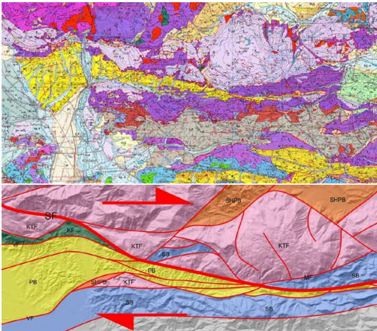
Slika 20: Izsek Osnovne geološke karte SFRJ v merilu 1:100000, list Ljubljana (Premru, 1983) in hipotetična in poenostavljena tektonska interpretacija; PB – Panonski bazen, VF – Viševski prelom, KF – kredni fliš, KTF – Krnski nariv, SB – Slovenski bazen (psevdoziljske plasti, ladinijski vulkaniti), MF – prelom Menine, SHPB – Slovensko-madžarski paleogenski bazen, SF – Savski prelom. Poenostavljeno po Premru (1983), Fodor et al. (1998), Vrabec (2001), Žalohar in Zevnik (2006).
