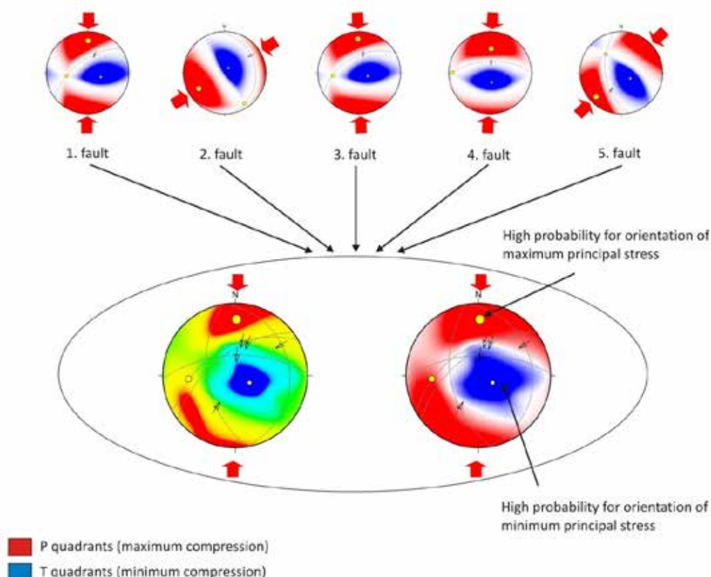
Slika 9: Primer paleonapetostne analize s programom T-TECTO 3.0 in metodo »Right Dihedra«.
