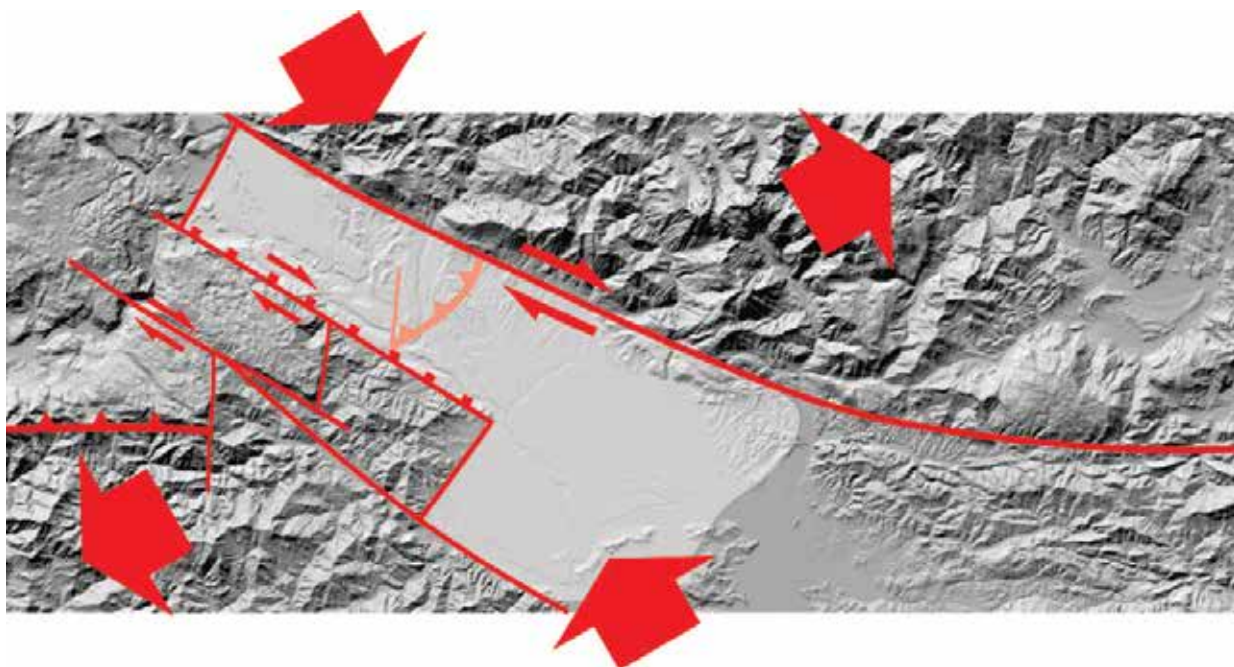
Slika 42: Nastanek normalnega preloma Krope in posledično Gorenjskega bazena.
