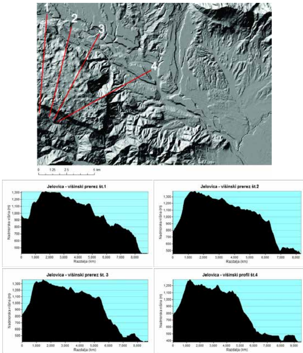
Slika 41: Višinski prerez čez Jelovico pri Kropi.
