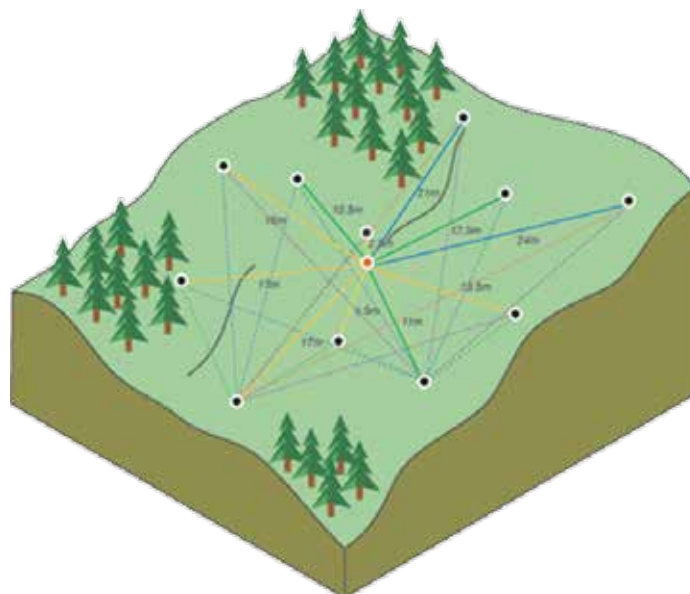
Slika 42: Pari razdalj med točkami.
