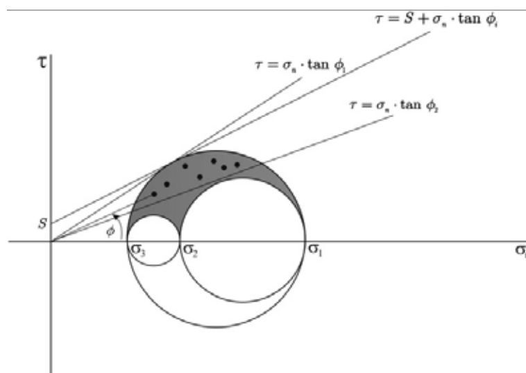
Slika 20: Mohrov diagram v treh dimenzijah prikazuje normalno in strižno napetost na prelomnice (črne 'Mohrove točke'). S_1 , S_2 in S_3 predstavljajo glavne napetosti, S pa je kohezija.
