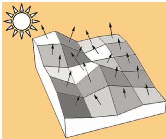
Slika 4: Shematičen prikaz analitičnega senčenja. Metoda predpostavlja vir osvetlitve na neskončni oddaljenosti ter konstantno vrednostjo azimuta in višinskega kota za vse celice v rastrskem sloju digitalnega modela reliefa.
