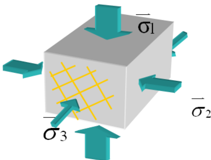
Slika 18: Glavne napetosti so med seboj pravokotne.
