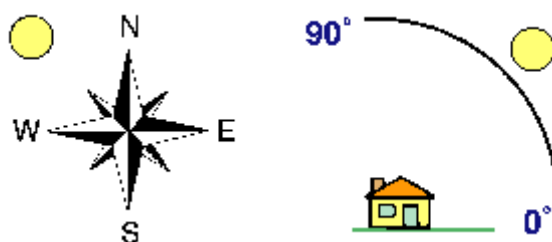
Slika 3: Ponazoritev azimuta in višinskega kota svetlobnega vira.
