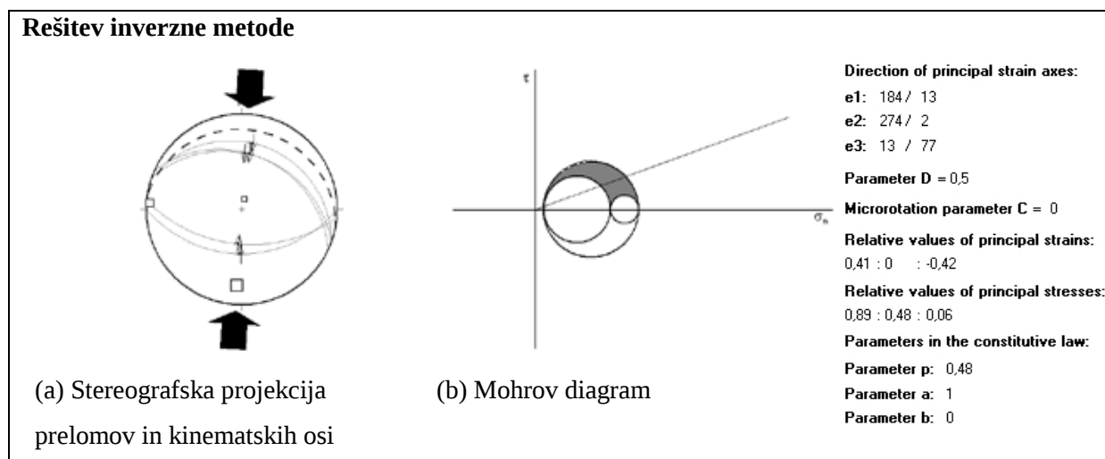
Slika 32: Rezultati kinematsko-napetostne analize prelomov pri Zadnjem vrhu.
