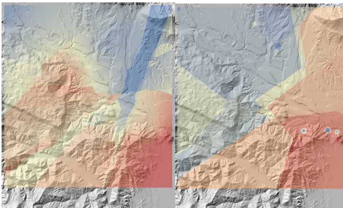
Slika 55: Primerjava rezultatov interpolacije po metodi kriging pred odstranitvijo točke (levo) in po odstranitvi točke (desno) v fazi N-S (zahodne točke).
