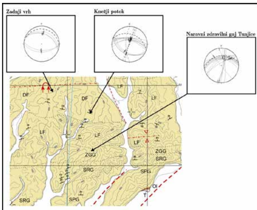
Slika 26: Geološka karta osrednjega dela južnega krila Tunjiške sinklinale ter stereografska projekcija prelomov pri Zadnjem vrhu, ob Knežjem potoku ter v Naravnem zdravilnem gaju Tunjice.
