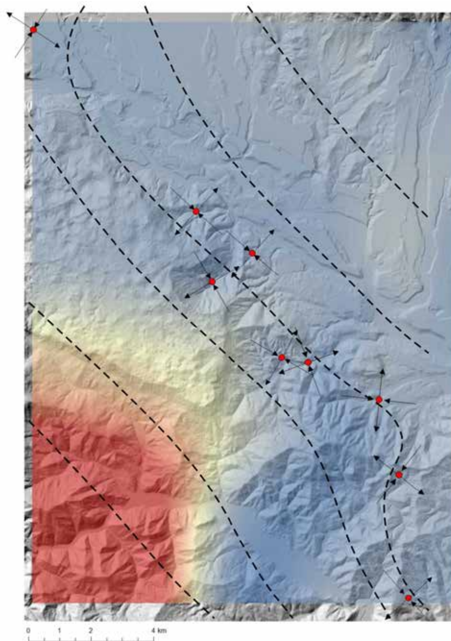
Slika 59: Trajektorije smeri maksimalne horizontalne kompresije v fazi kompresije NW-SE in ekstenzije (zahodne točke).
