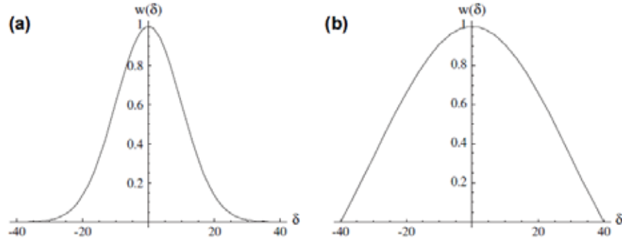
Slika 24: Utežna funkcija w(\delta) za dve različni vrednosti parametra s : V a) primeru je D = 40^\circ , v b) primeru pa je D = 30^\circ
