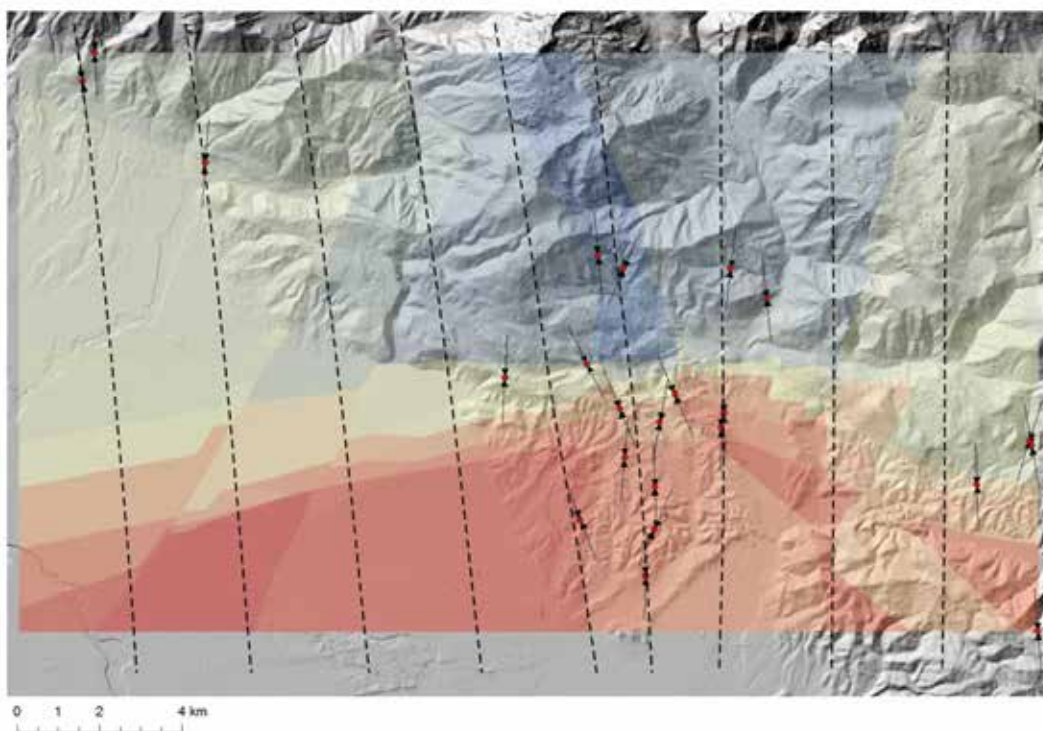
Slika 60: Trajektorije smeri maksimalne horizontalne kompresije v fazi N-S (vzhodne točke)
