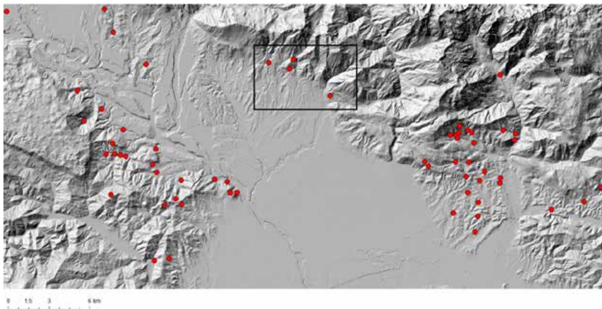
Slika 43: Razporeditev točk, na katerih so bile izvedene meritve.
