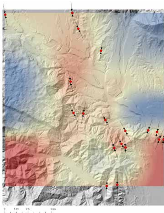
Slika 58: Azimuti maksimalne horizontalne kompresije v fazi N-S (zahodne točke)
