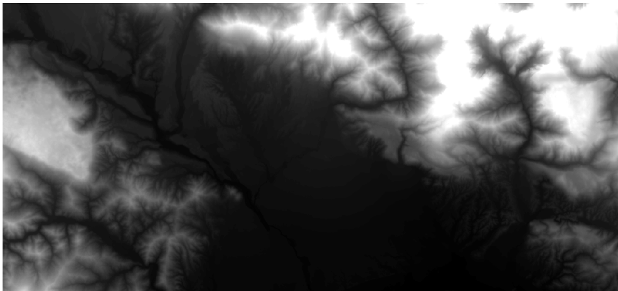
Slika 2: Zapis DMV, kjer paleta sivih vrednosti ustreza različnim vrednostim nadmorskih višin. Prikazuje območje med Kropo in Kamnikom.
