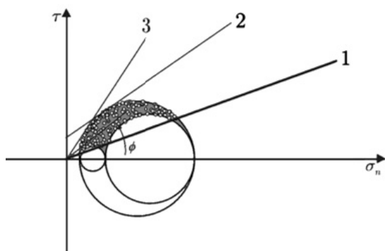
Slika 22: Prelamljanje nastopi takrat, ko se Mohrova krožnica s središčem 1/2(\sigma_1 + \sigma_2) in premerom (\sigma_1 - \sigma_3) dotakne krivulje 2 na sliki. To krivuljo imenujemo Mohrova ovojnica, saj jo dobimo kot ovojnico Mohrovih krožnic, ki ustrezajo prelamljanju pri različnih napetostih.
