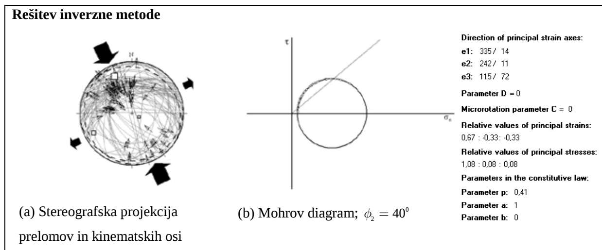
Slika 28: Rezultati kinematsko-napetostne analize prelomov v okolici krajev Viševca in Vrhovlje – prelamljanje v času, ko so bile plasti še v horizontalni do subhorizontalni legi.
