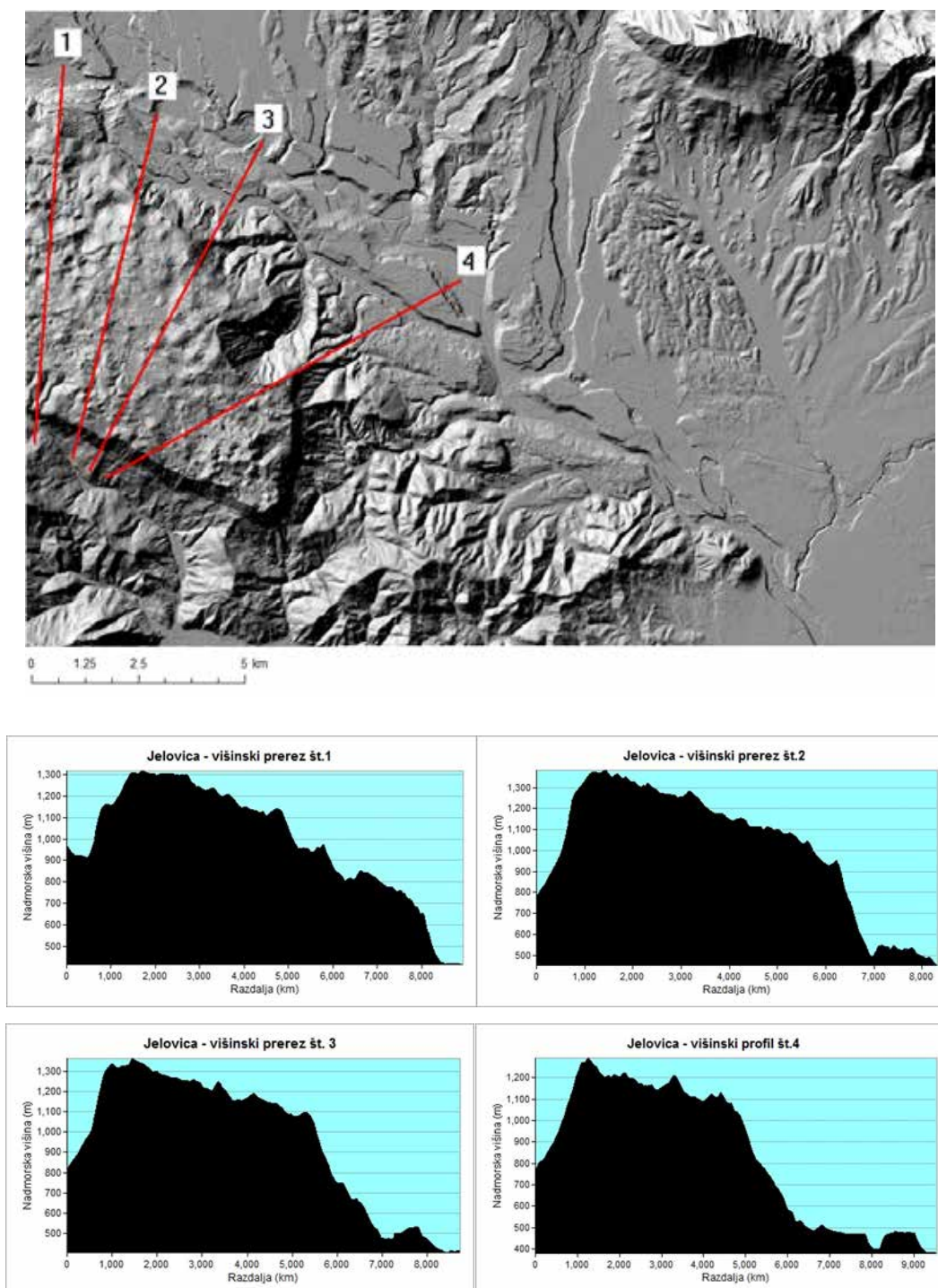
Slika 8: Višinski prerez skozi Jelovico.
