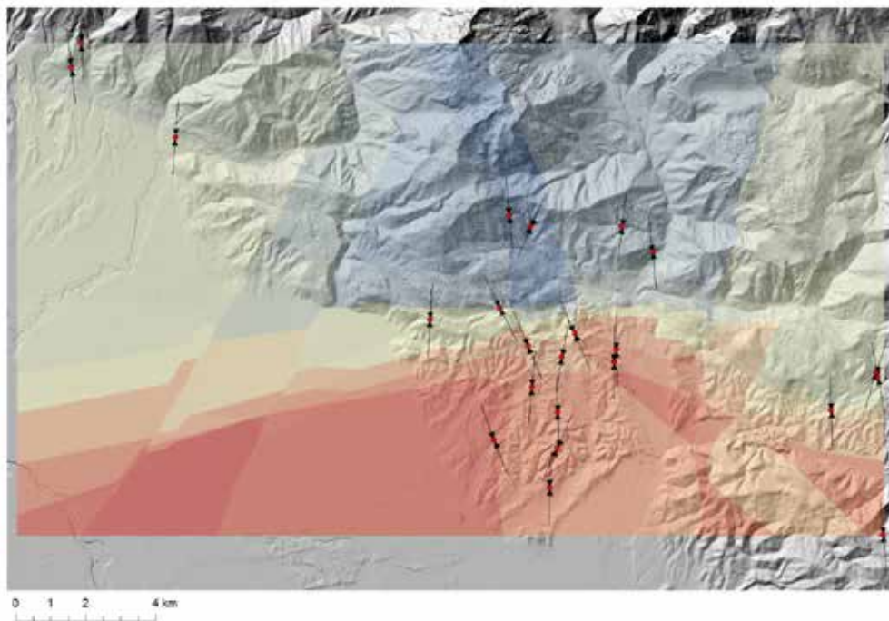
Slika 57: Azimuti maksimalne horizontalne kompresije v fazi N-S (vzhodne točke)
