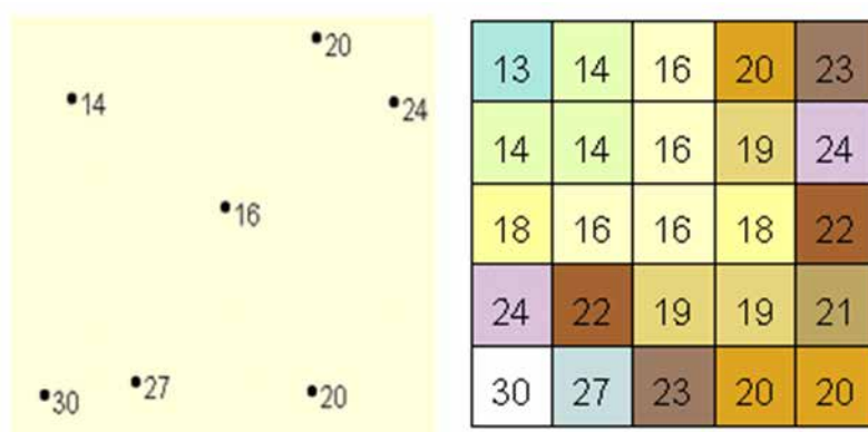
Slika 35: Vrednosti vzorčnih točk (levo) in iz njih generiran rastrski sloj (desno). Neznane vrednosti vmesnih točk vrednosti predvidimo z uporabo matematičnih algoritmov, ki za njihovo določitev uporabijo vrednosti znanih bližnjih točk.
