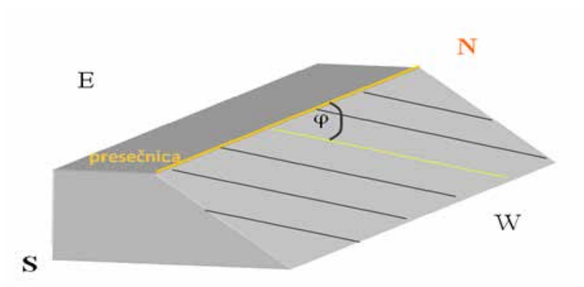
Slika 14: Merjenje naklona drsnih lineacij.
