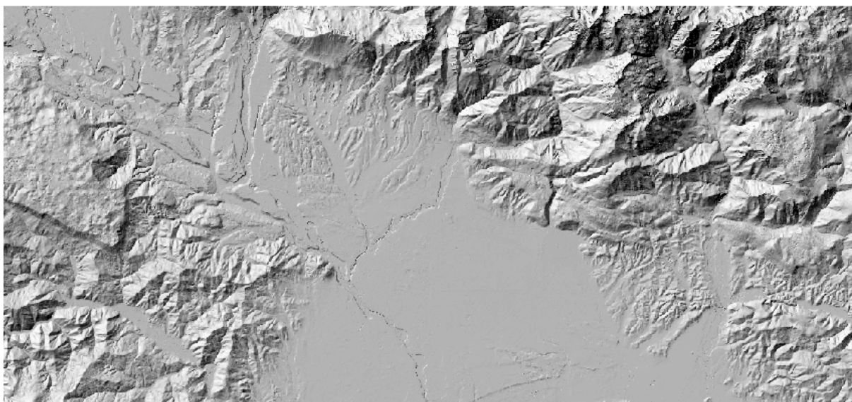
Slika 5: Senčen digitalni model reliefa. Azimut Sonca znaša 315^\circ , višinski kot pa 45^\circ .
