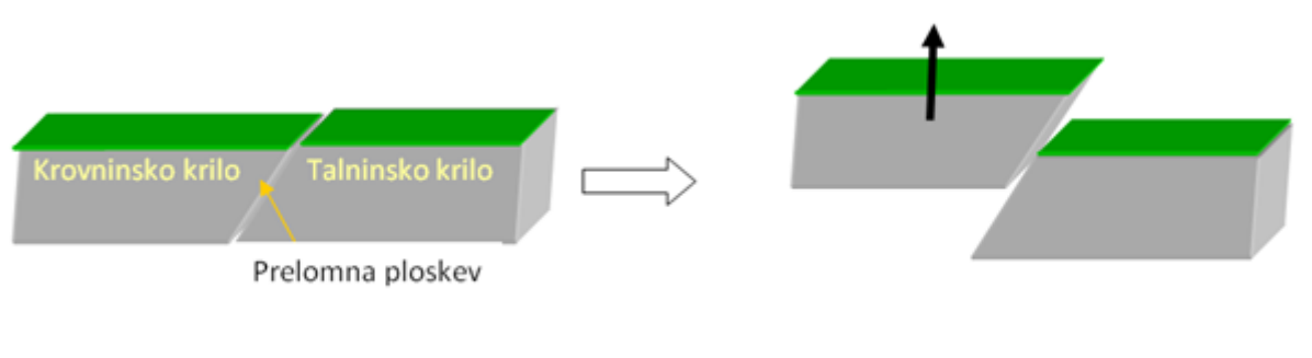
Slika 11: Reverzni prelom: Krovninsko krilo (nad prelomno ploskvijo) se je relativno dvignilo glede na talninsko (pod prelomno ploskvijo).
