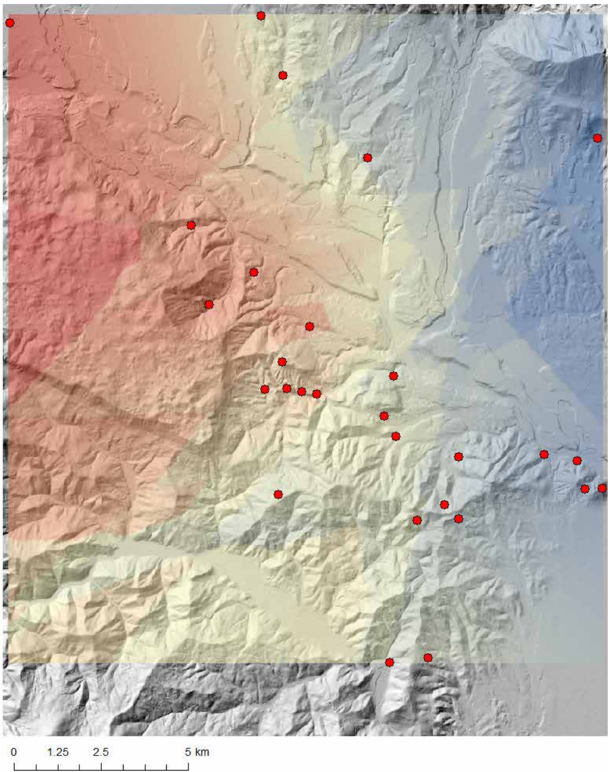
Slika 47: Interpolirana ploskev z metodo zlepkov za fazo ekstenzije za zahodne točke.
