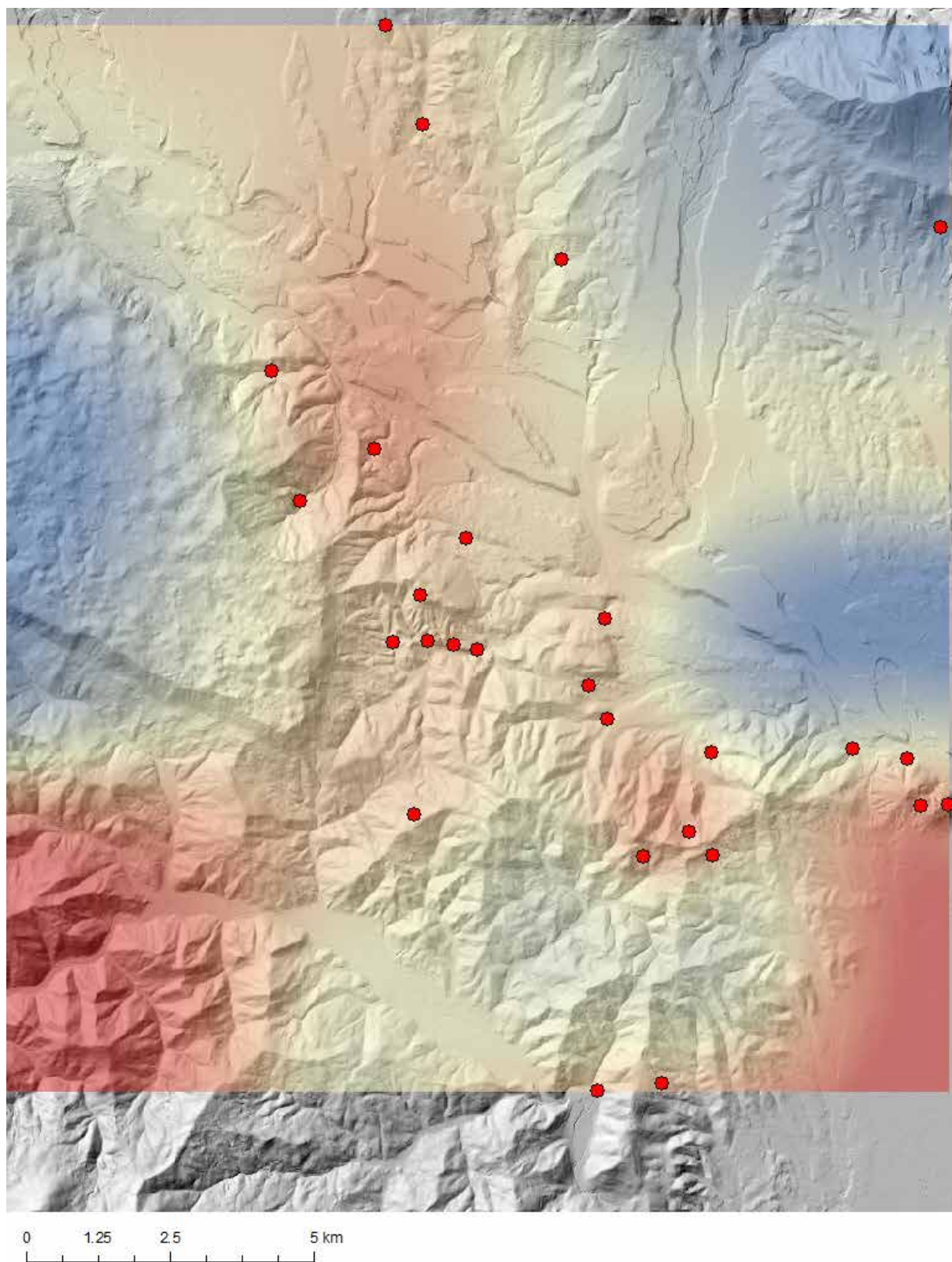
Slika 49: Interpolirana ploskev z metodo zlepkov za fazo N-S za zahodne točke.
