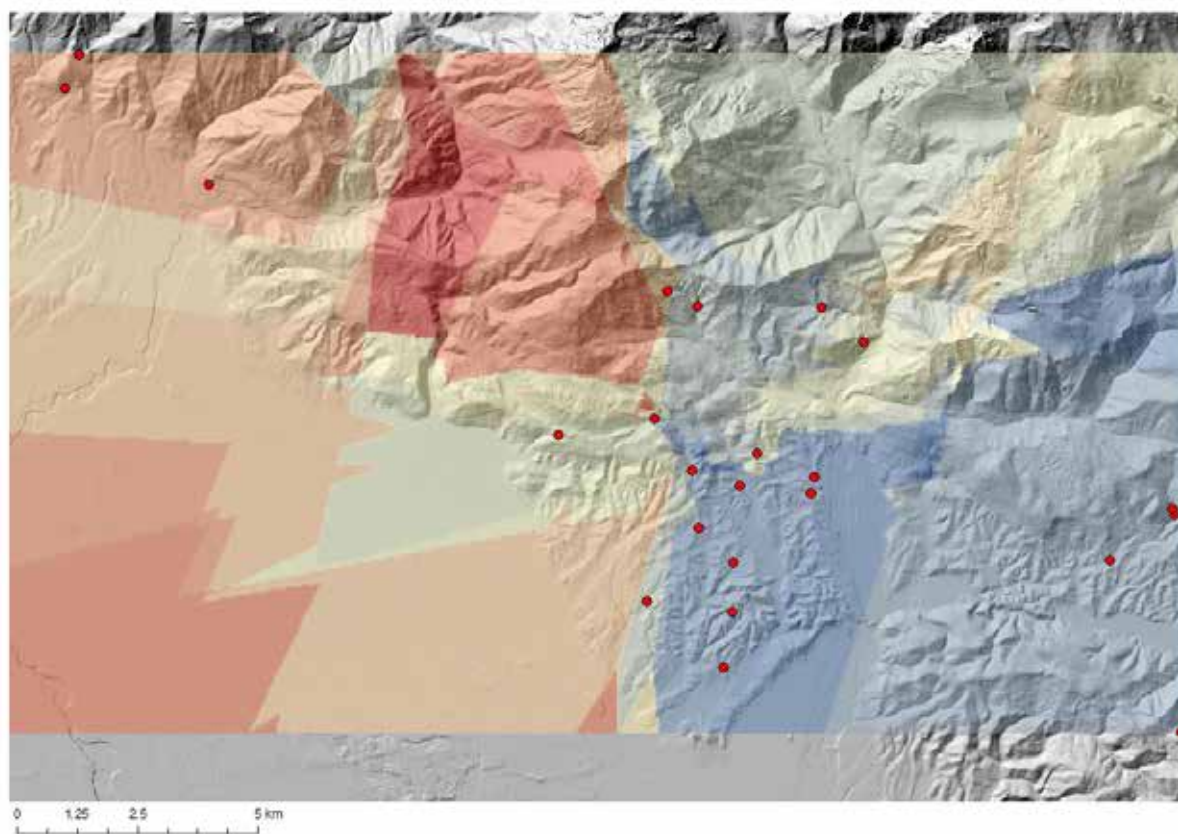
Slika 51: Interpolirana ploskev z metodo kriging za fazo NW-SE za vzhodne točke.
