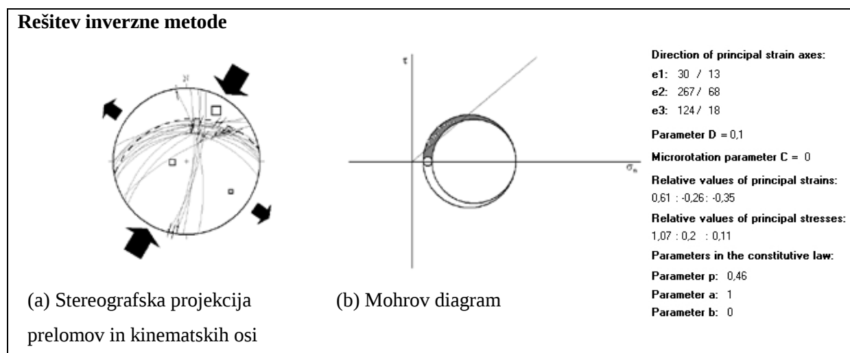
Slika 34: Rezultati kinematsko-napetostne analize prelomov v peskokopu južno od cerkve sv. Ane (Naravni zdravilni gaj Tunjice).
