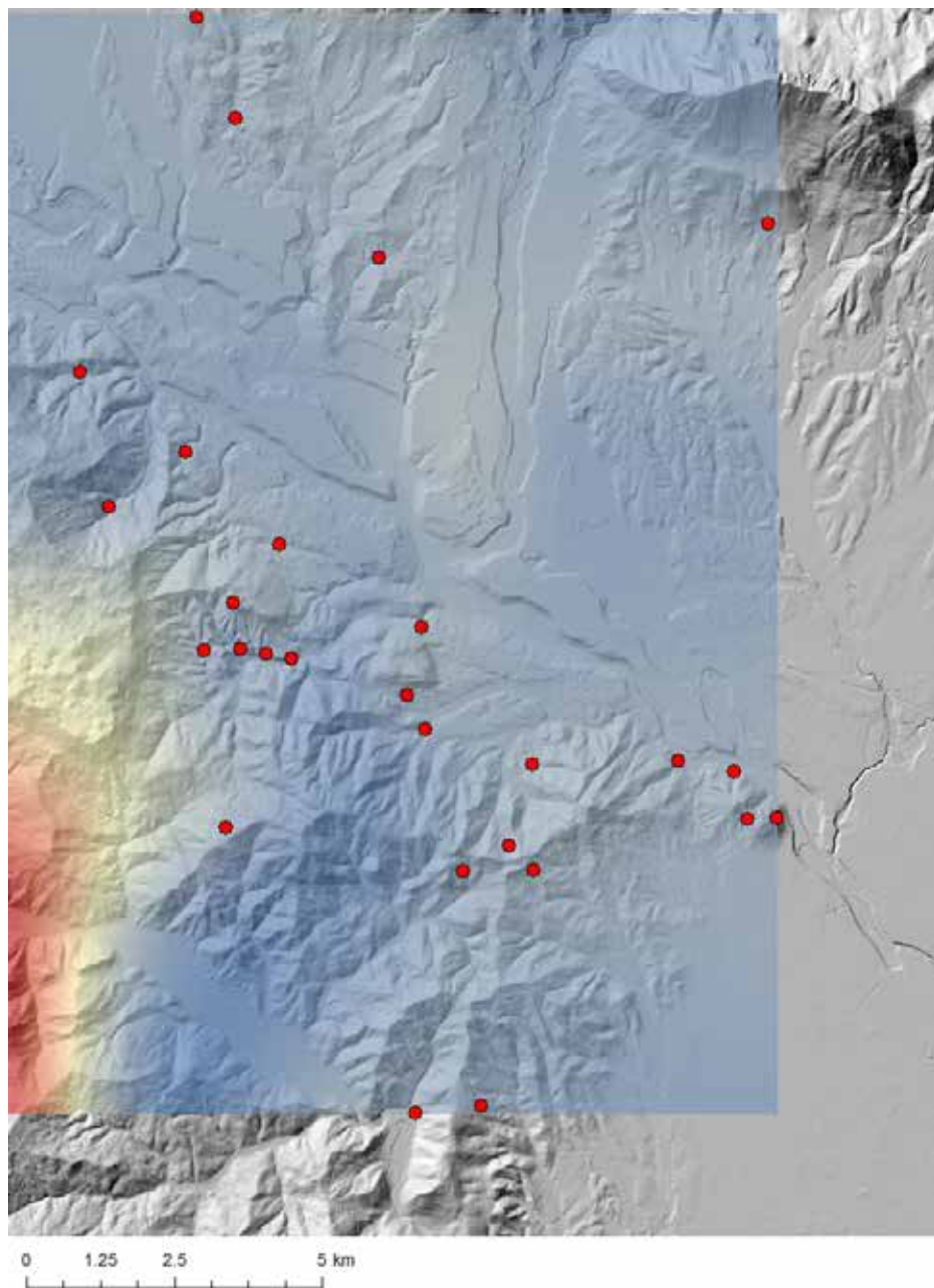
Slika 46: Interpolirana ploskev z metodo kriging za fazo ekstenzije za zahodne točke.
