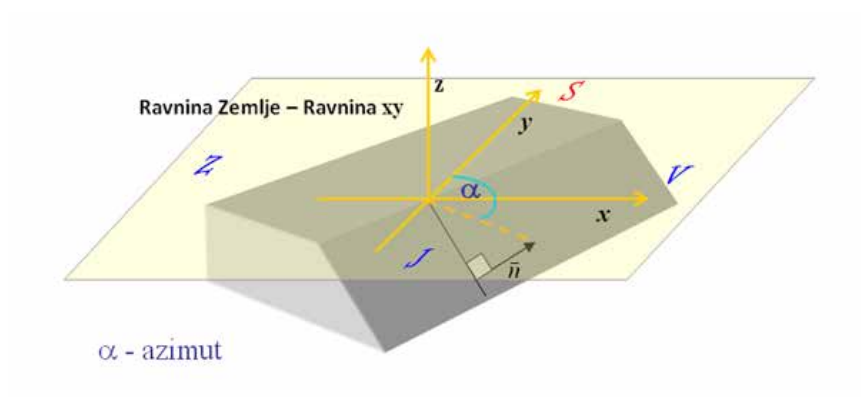
Slika 16: Azimut je definiran kot kot med osjo y in projekcijo normale preloma (pravokotnica na ravnino preloma)
