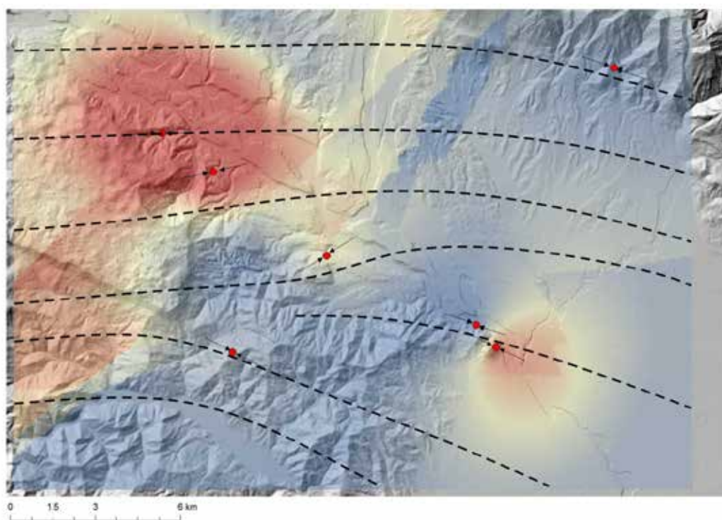
Slika 63: Trajektorije smeri maksimalne horizontalne kompresije v fazi W-E
