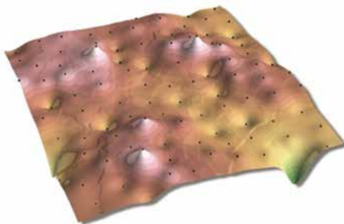
Slika 39: Ploskev, pridobljena z metodo utežne obratne razdalje.
