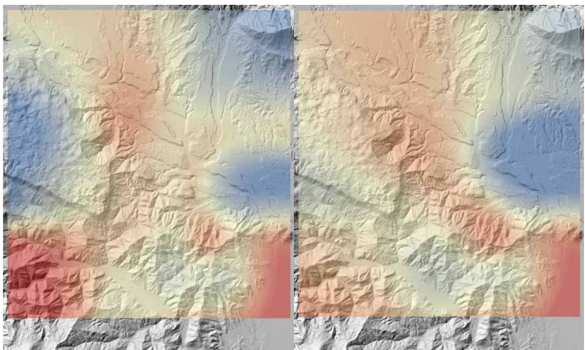
Slika 54: Primerjava rezultatov interpolacije po metodi zlepkov pred odstranitvijo točke (levo) in po odstranitvi točke (desno) v fazi N-S (zahodne točke).
