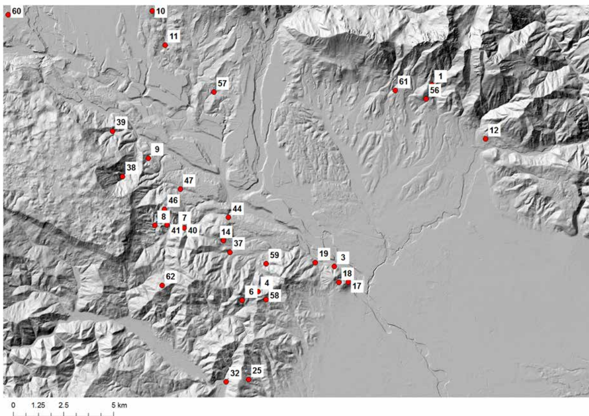
Slika 44: Razporeditev in gostota točk na zahodnem delu obravnavanega območja
