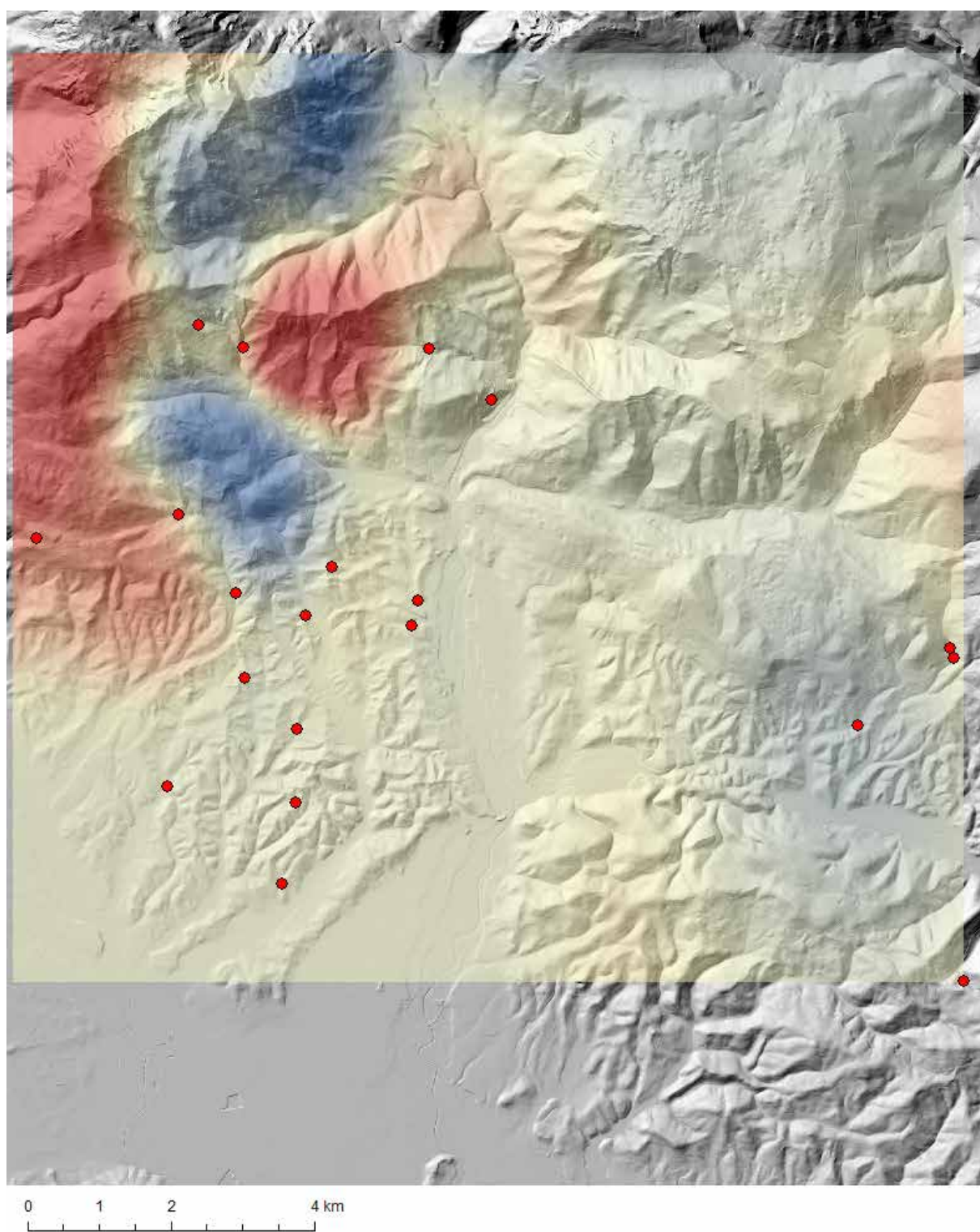
Slika 52: Interpolirana ploskev z metodo zlepkov za fazo NW-SE za vzhodne točke.
