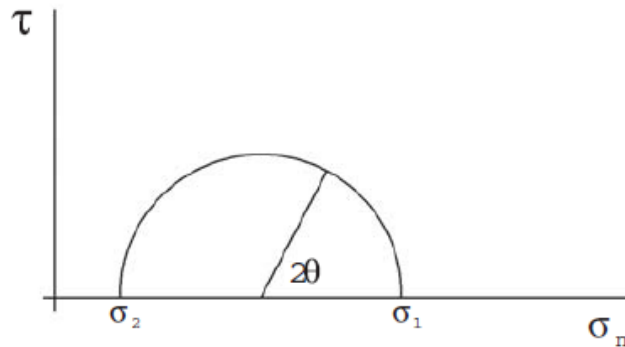
Slika 19: Mohrov diagram v dveh dimenzijah. Predznak strižne napetosti vpliva le na njeno smer, zato nas pri Mohrovi konstrukciji zanima le velikost strižne napetosti t .
