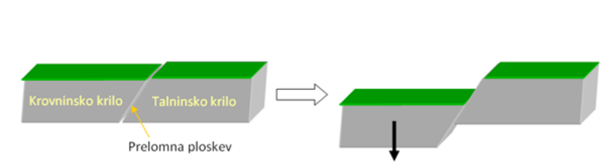
Slika 10: Normalni prelom: Krovninsko krilo (nad prelomno ploskvijo) se je relativno spustilo glede na talninsko (pod prelomno ploskvijo).
