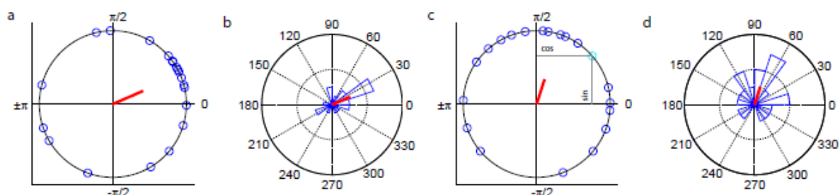
Slika 56: Predstavitev vektorskih podatkov na kotni skali.
