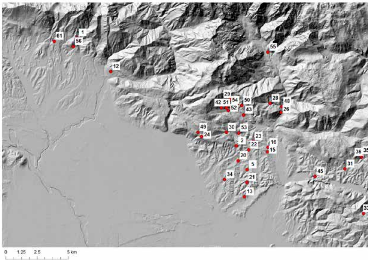
Slika 45: Razporeditev in gostota točk na vzhodnem delu obravnavanega območja
