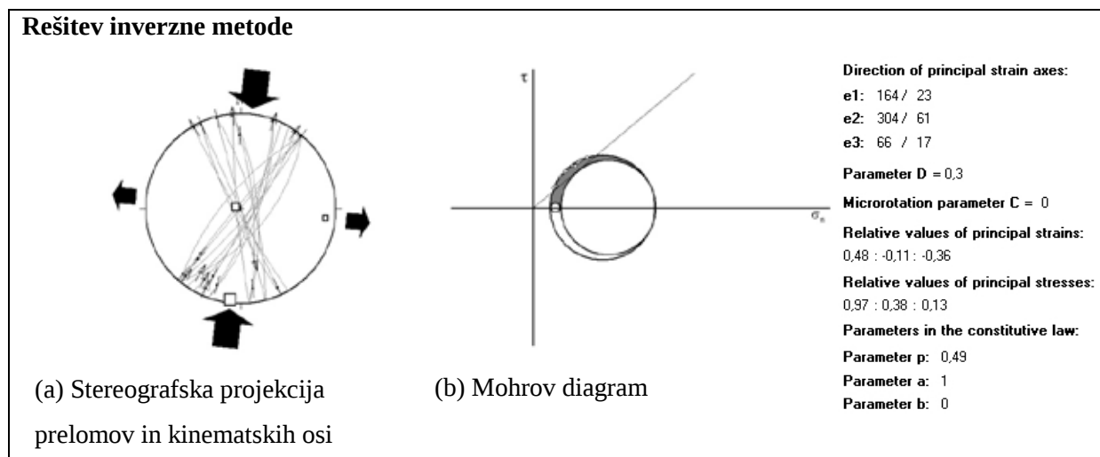
Slika 31: Rezultati kinematsko-napetostne analize prelomov ob cesti Laniše–Stranje.
