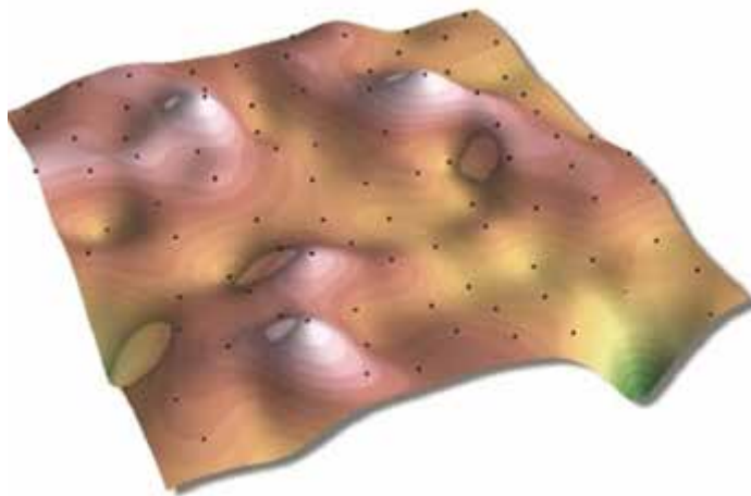
Slika 40: Ploskev, pridobljena z metodo zlepkov.
