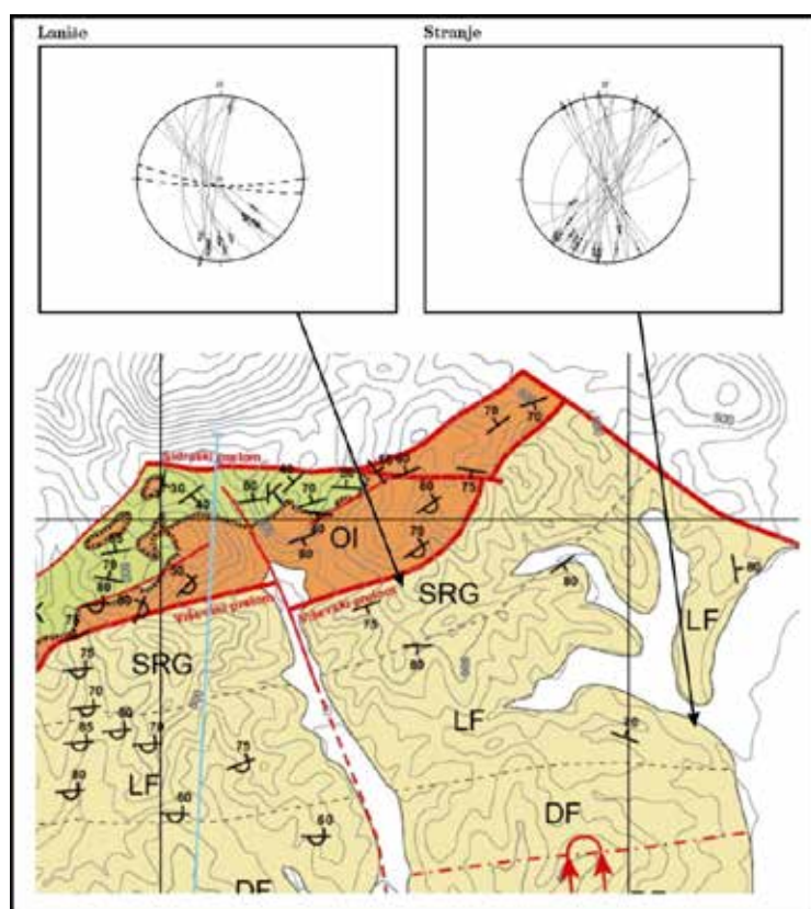
Slika 27: Geološka karta vzhodnega dela severnega krila Tunjiške sinklinale ter stereografska projekcija prelomov pri Lanišah in Stranjah.
