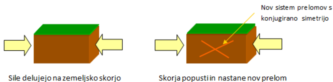
Slika 9: Shema procesa prelamljanja zemeljske skorje.
