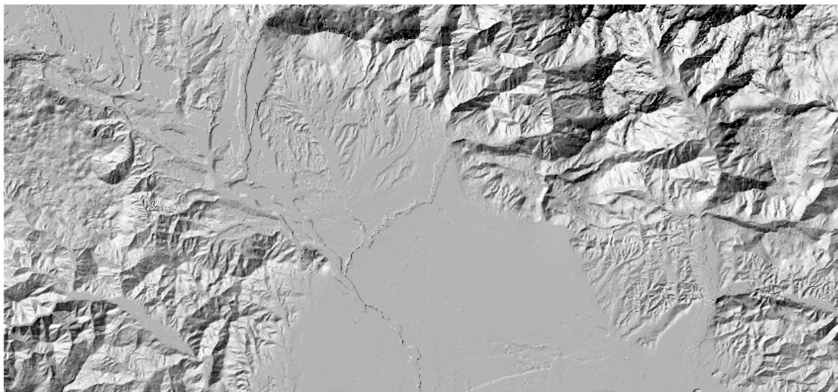
Slika 6: Senčen digitalni model reliefa. Azimut Sonca znaša 135^\circ , višinski kot pa 45^\circ .
