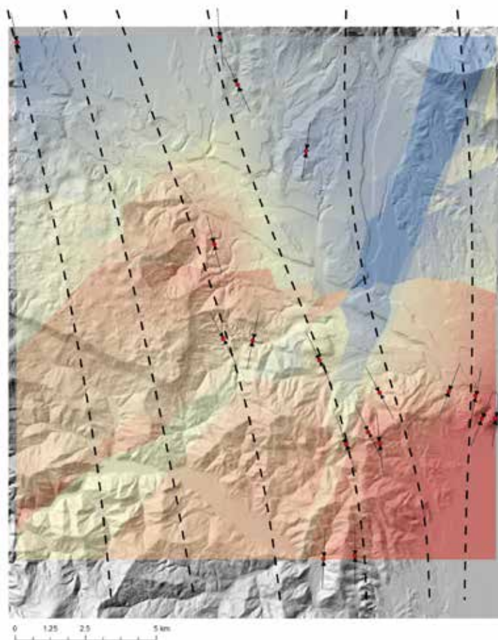
Slika 61: Trajektorije smeri maksimalne horizontalne kompresije v fazi N-S (zahodne točke).
