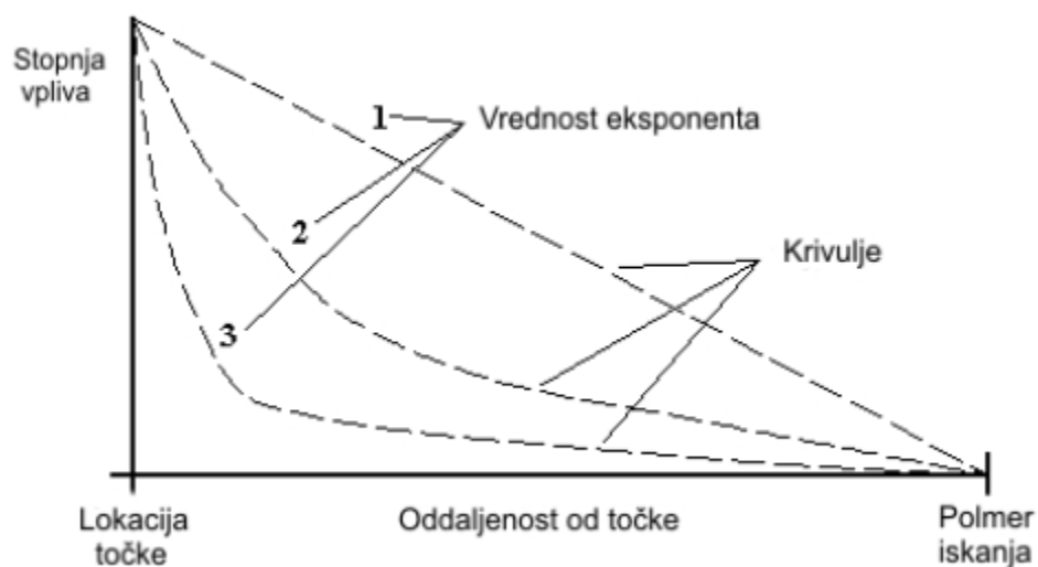
Slika 38: Vpliv utežne potence.
