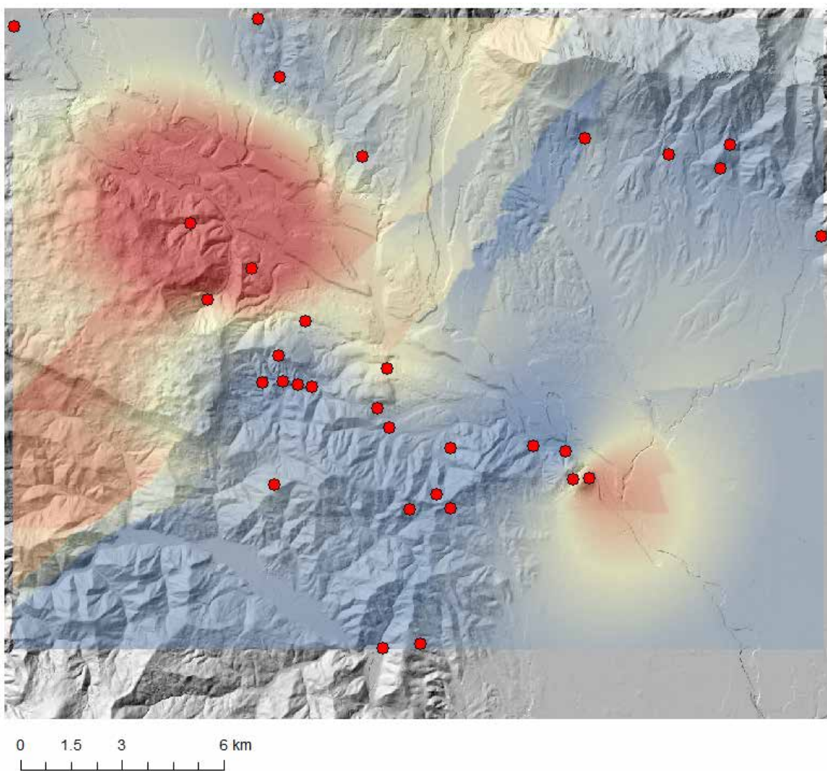
Slika 48: Interpolirana ploskev z metodo kriging za fazo W-E za zahodne točke.
