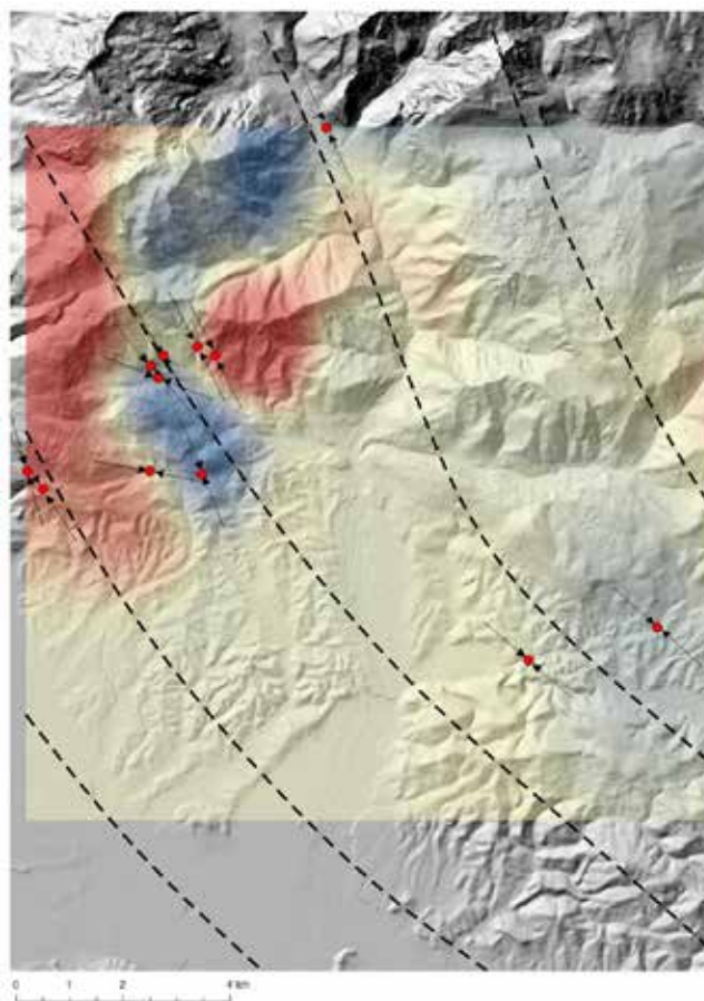
Slika 62: Trajektorije smeri maksimalne horizontalne kompresije v fazi NW-SE (vzhodne točke)
