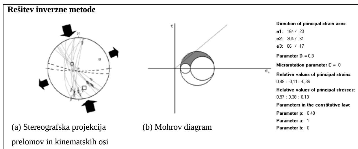
Slika 30: Rezultati kinematsko-napetostne analize prelomov pri Lanišah.
