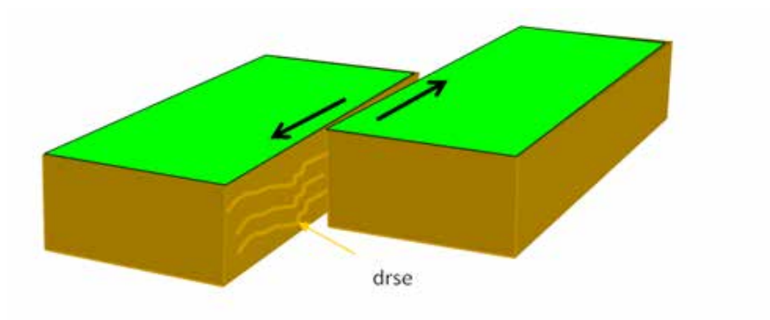
Slika 13: Nastanek drsnih lineacij.
