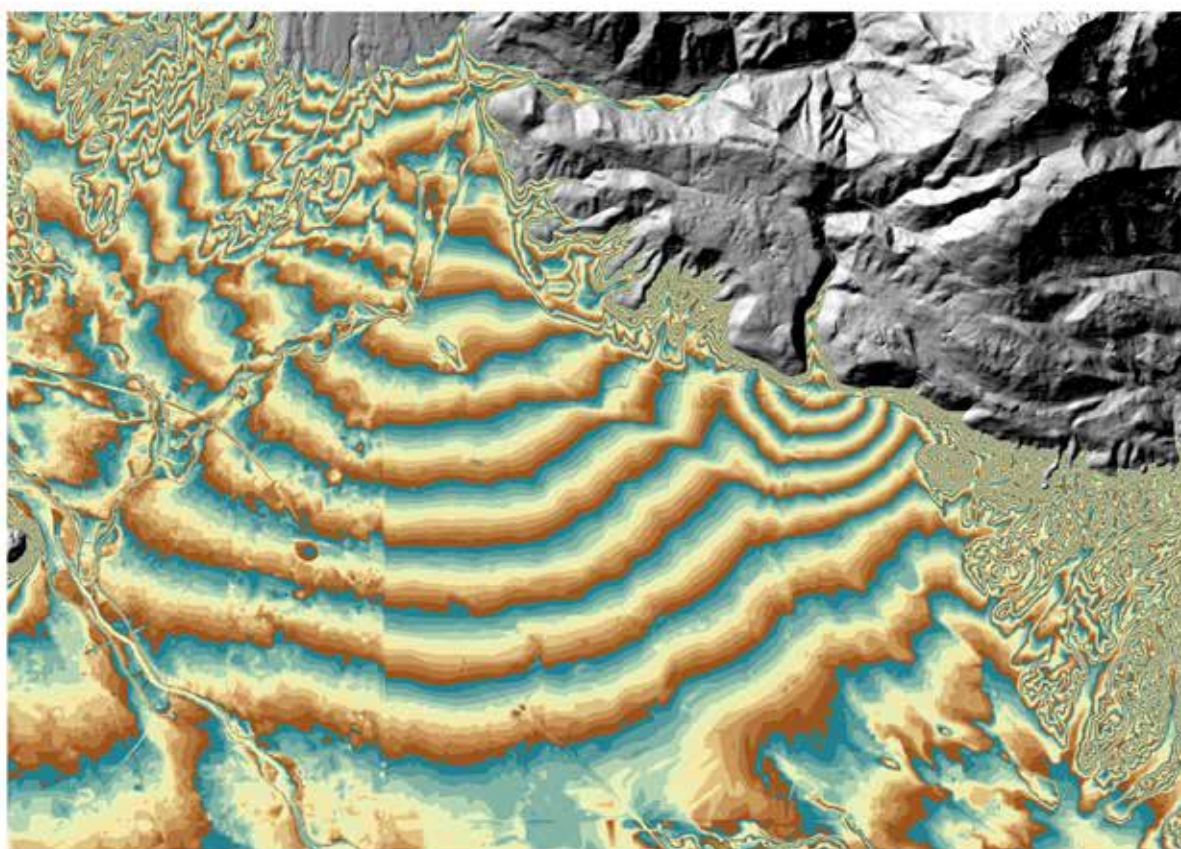
Slika 7: Prikaz digitalnega modela reliefa z metodo bipolarnega diferenciranja.
