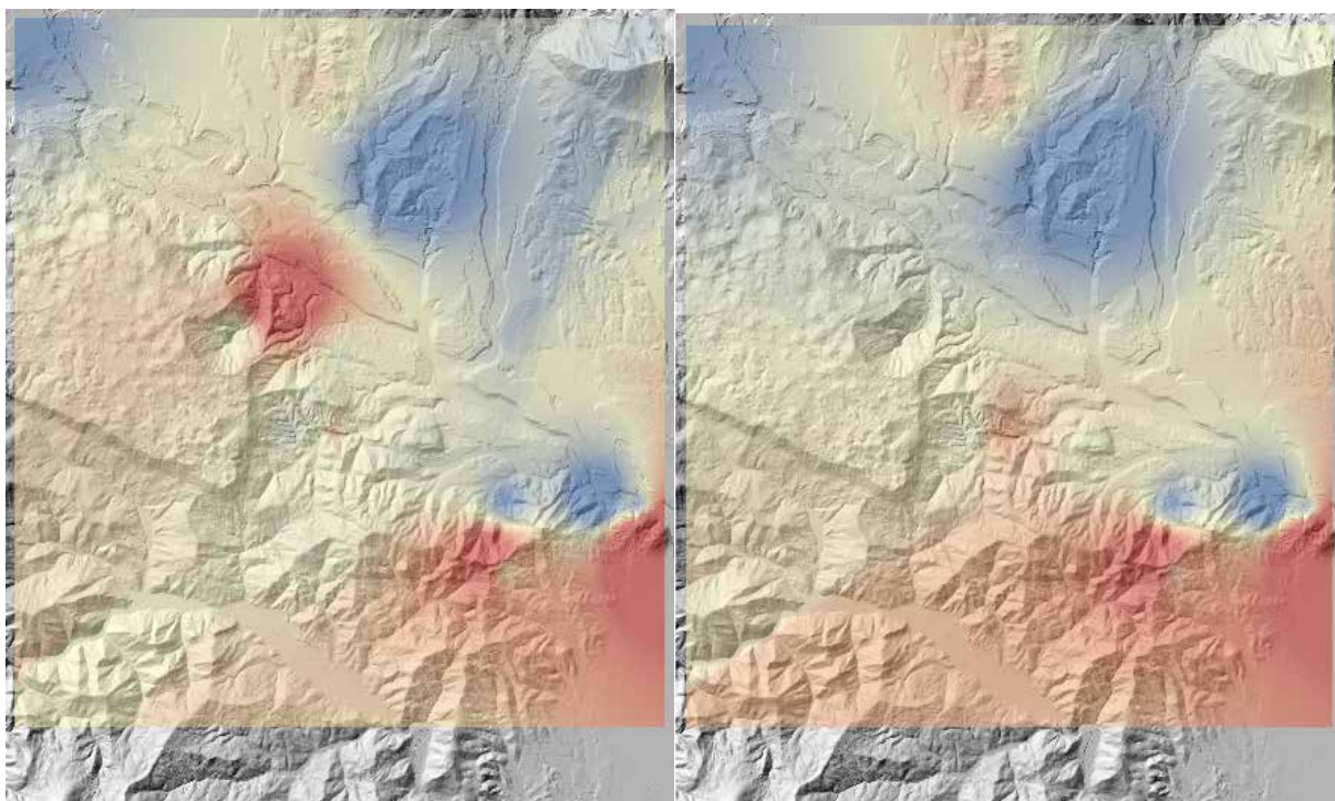
Slika 53: Primerjava rezultatov interpolacije po metodi utežne obratne razdalje pred odstranitvijo točke (levo) in po odstranitvi točke (desno) v fazi N-S (zahodne točke).
