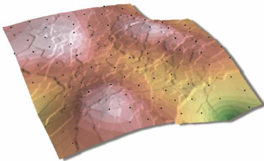
Slika 41: Ploskev, pridobljena z metodo kriging.
