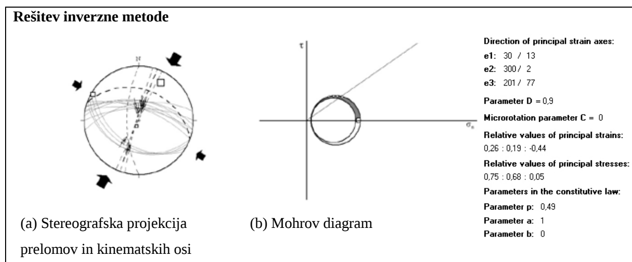
Slika 33: Rezultati kinematsko-napetostne analize prelomov ob Knežjem potoku.
