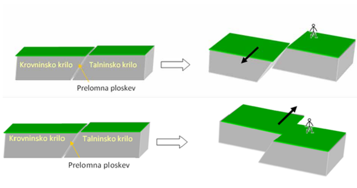
Slika 11: Reverzni prelom: Krovninsko krilo (nad prelomno ploskvijo) se je relativno dvignilo glede na talninsko (pod prelomno ploskvijo).
