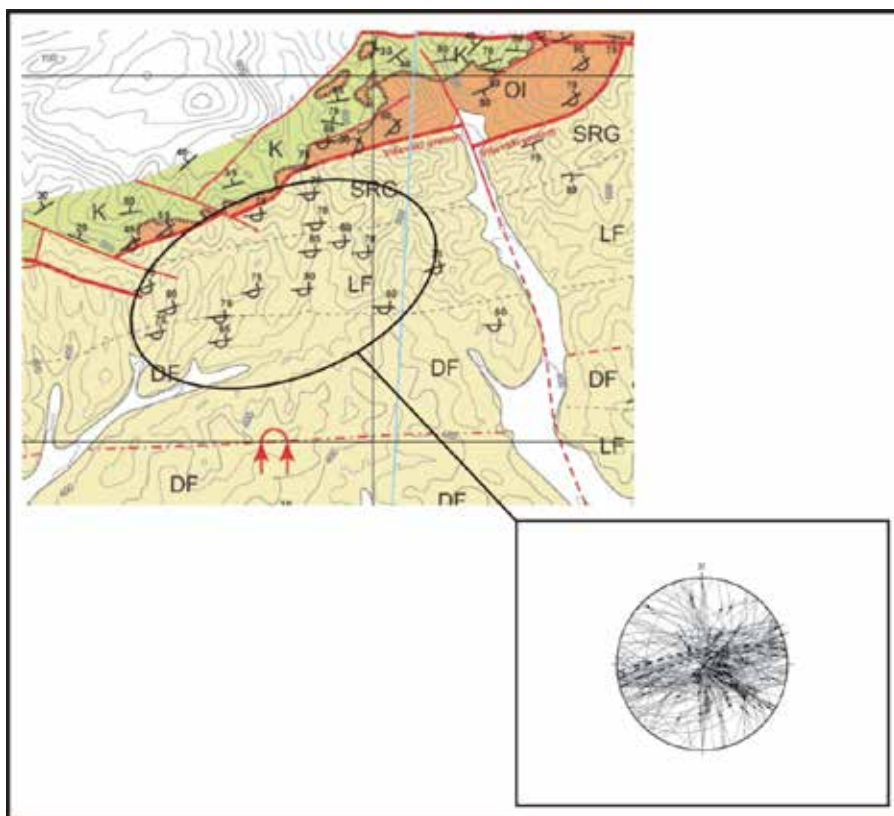
Slika 25: Geološka karta severnega krila Tunjiške sinklinale ter stereografska projekcija prelomov in povprečnega vpada plastnatosti.
