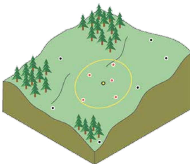
Slika 37: Vpliv števila sosednjih točk in polmera območja interpolacije.
