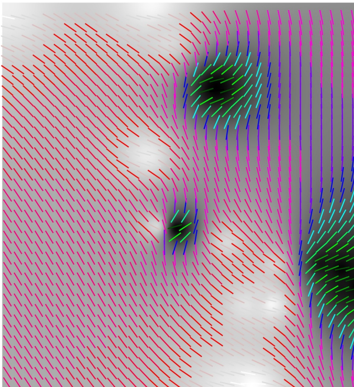
Slika 64: Interpolirano vektorsko polje.
