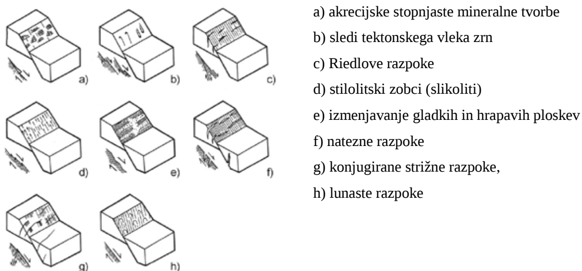
Slika 15: Kinematski indikatorji – obstaja več različnih oblik kinematskih indikatorjev, ki jih uporabljamo kot kriterij za določanje smeri premika
