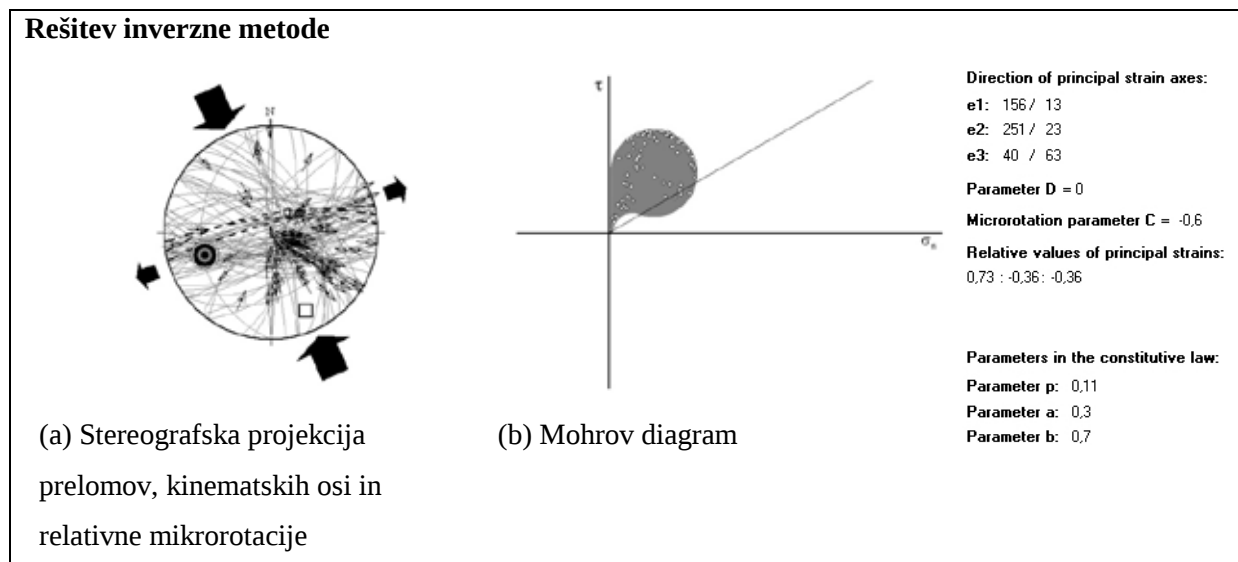
Slika 29: Rezultati kinematsko-napetostne analize prelomov v okolici krajev Viševca in Vrhovlje – prelamljanje po nagibu plasti v današnji položaj zaradi gubanja Tunjiške sinklinale.
