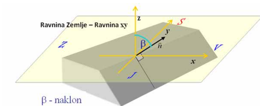
Slika 17: Naklon je definiran kot kot med prelomno ploskvijo in ravnino xy, oz. kot kot med normalo in osjo z. Zavzame lahko vrednosti od 0 do 90°.
