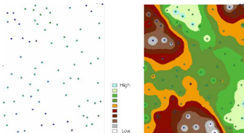
Slika 36: Točke s podatkom o višini ter interpolirana ploskev.
