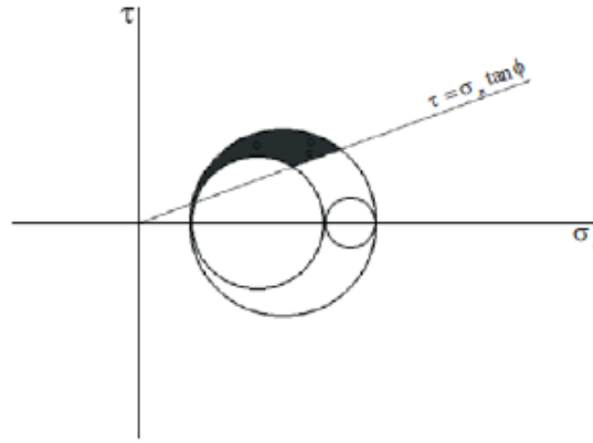
Slika 21: Do premika na neki planarni diskontinuiteti pride, če pripadajoča točka na Mohrovem diagramu, ki predstavlja stanje napetosti na tej diskontinuiteti, leži nad premico \tau = \sigma_n \tan f (Amontonov zakon). Točka mora torej ležati znotraj potemnjene območja.
