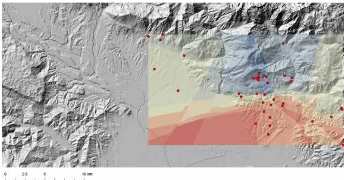
Slika 50: Interpolirana ploskev z metodo kriging za fazo N-S za vzhodne točke.
