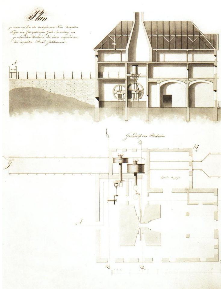
Slika 13: Načrt prenove plavža na Javorniku
