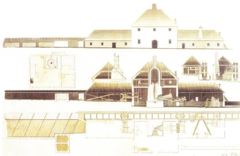
Slika 11: Prikaz delovanja Zoisovega plavža na Javorniku
