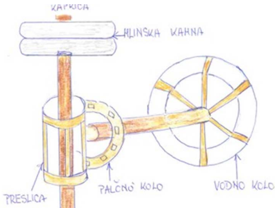
Slika 10: skica delovanja vodnega pogona
